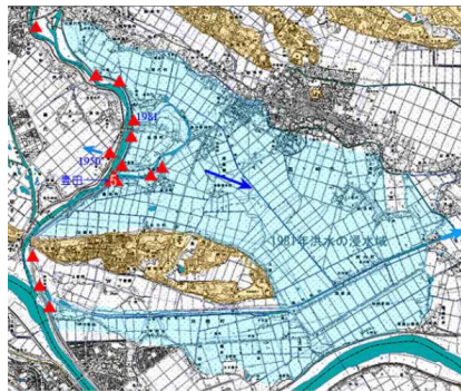
図 10 小貝川の堤防決壊箇所(1742 年以降)
