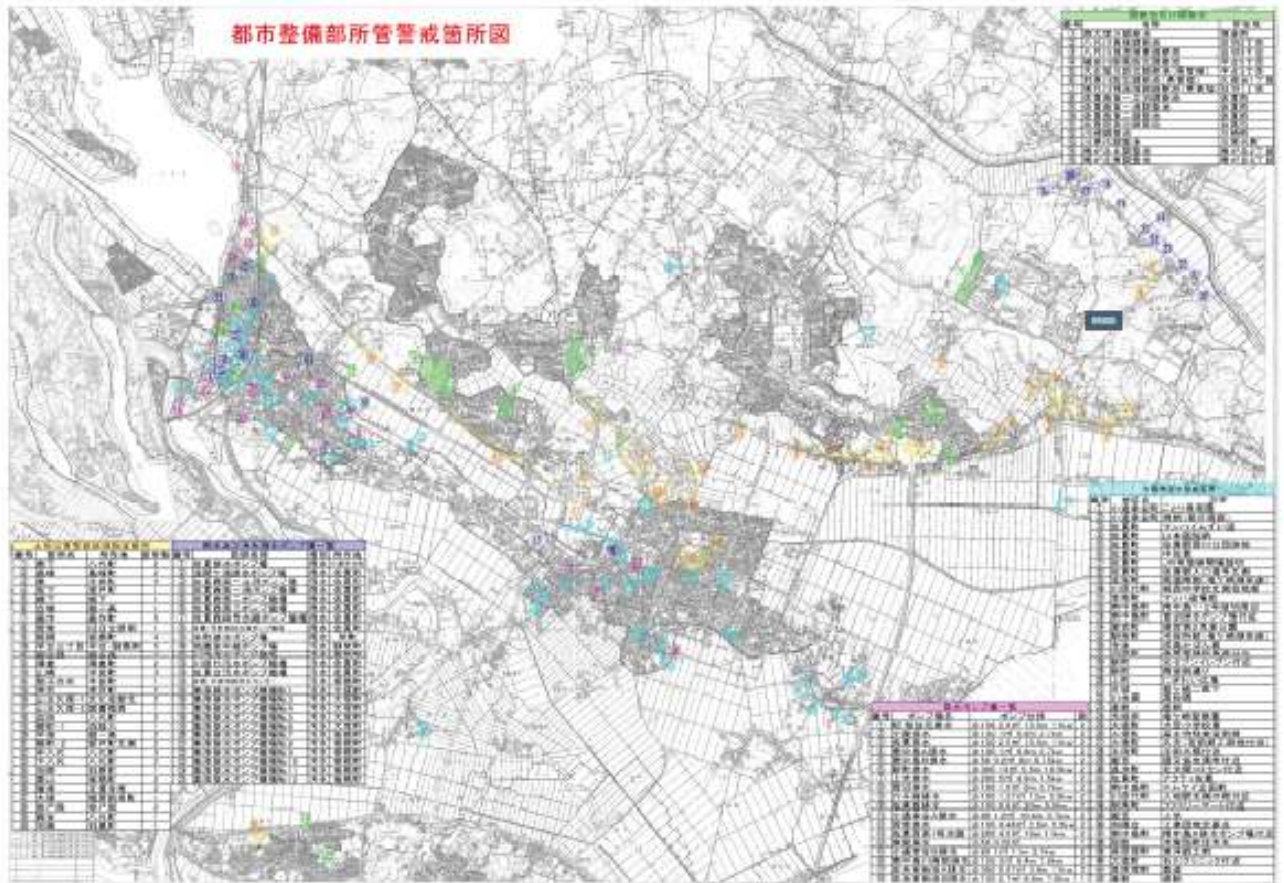
(図 5) 都市整備部所管警戒箇所図
