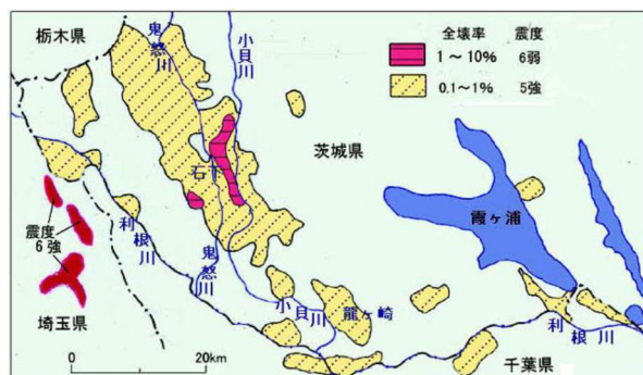
(図6) 1923年関東大震災による住家全壊
