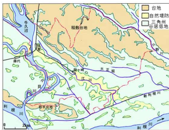
(図 1)：地形分類図
