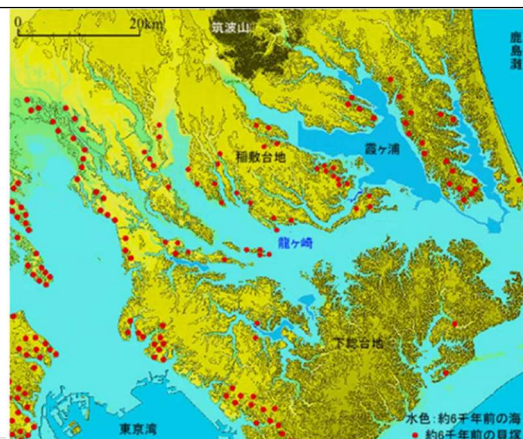
(図 2) 約 6 千年前の関東平野
