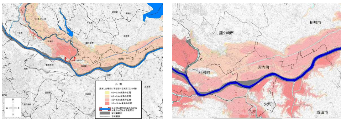
(左：図 3) 利根川水系小貝川洪水浸水想定区域図
